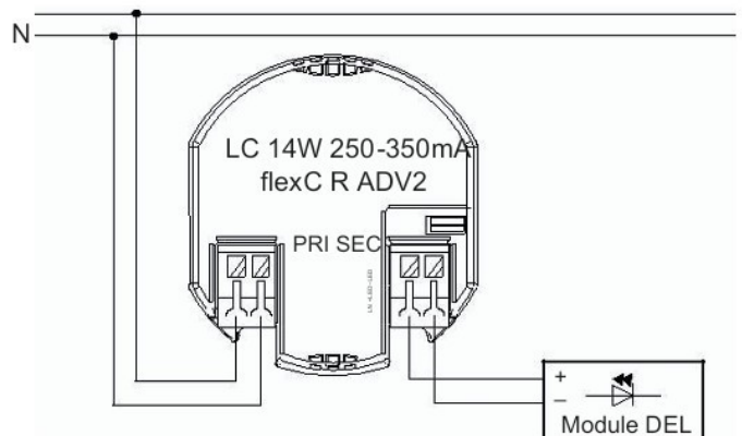
SCHÉMA D'INSTALLATION
