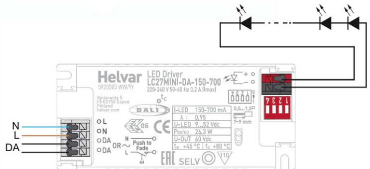
SCHÉMA D'INSTALLATION
