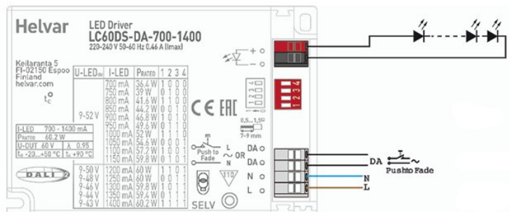
SCHÉMA D'INSTALLATION
