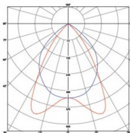
Courbe photométrique TRU LED 3360 lm 28W
